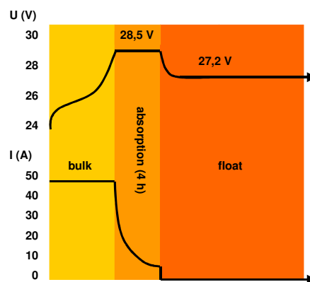
Ladekennlinie
